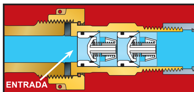
Presión de agua negativa – la válvula cierra
