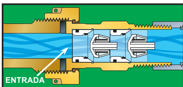
Presión de agua positiva – la válvula abre
