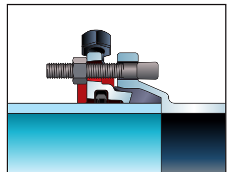
3"-12" SO-EZ Gasket
