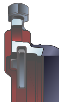
3"-12" SO-EZ Gasket
