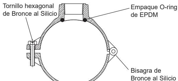
Estilo A (Diseño Abisagrado)
