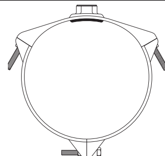
Estilo C - 3 Piezas (Diseño Atornillado)
