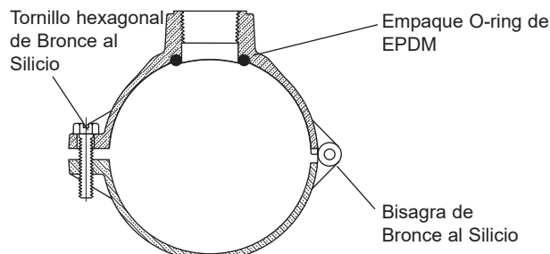
Estilo A (Diseño Abisagrado)
